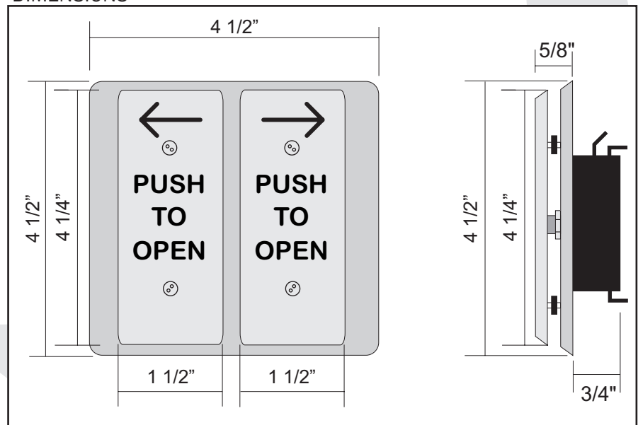
DIMENSIONS
